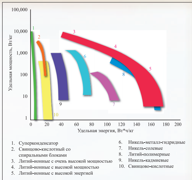
Сравнение удельной энергии и мощности среди различных видов аккумуляторных батарей
